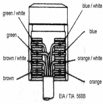
EIA/TIA 568B
