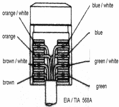
EIA/TIA 568A
